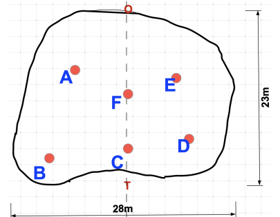
TROU N°15
