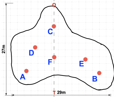
TROU N°16
